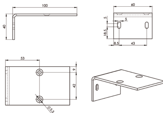
Guide rail (7-303770-0000)
